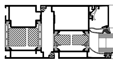
Schüco ADS 75 HD.HI, Horizontalschnitt, Maßstab 1:2 Schüco ADS 75 HD.HI, horizontal section detail, scale 1:2
